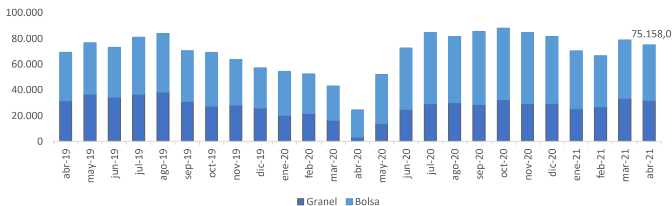
Gráfico N°5. Consumo de Cemento Portland en toneladas. Provincia de Santa Fe
